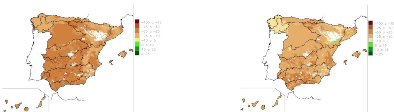
Escenarios de emisiones A2 2071-2100 sobre 1961-1990
